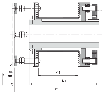
.../SI/ML (с длинной ступицей)
