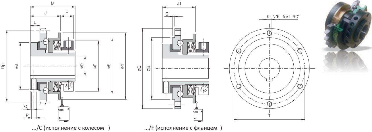
.../C (исполнение с колесом ) .../F (исполнение с фланцем )
