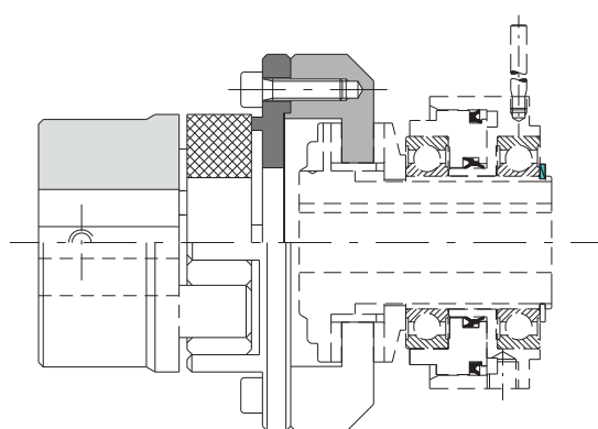
Модель DSF/TF/AP с эластичной кулачковой муфтой GAS для устранения больших смещений.
