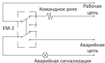
Переключатель с двумя контактами (ЕМ2).
