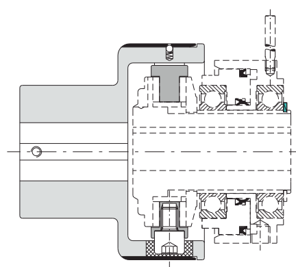
Модель DSF/TF/AP с компактной эластичной муфтой GEC для простого техобслуживания без удаления муфты
