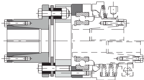
DSS/SG модель с металлической дисковой муфтой GTR/D, с одним изгибом для применения, где требуется жесткость на кручение
