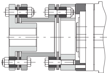
DSS/SG модель с металлической дисковой муфтой GTR/D, жесткой на кручение, с двойным нагибом, когда требуется жесткость на кручение имеет способность демпфировать радиальное смещение
