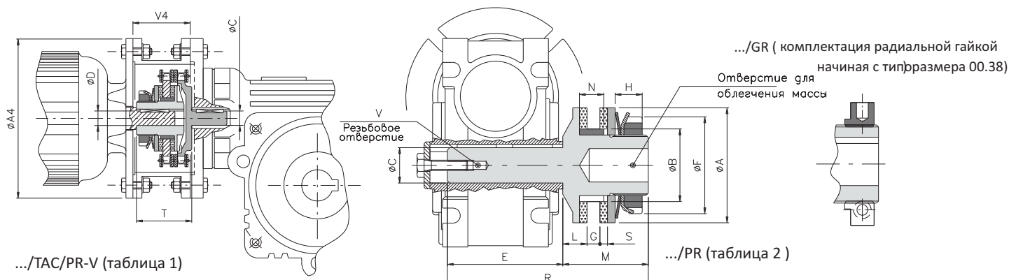
ГАБАРИТНО-ПРИСОЕДИНИТЕЛЬНЫЕ РАЗМЕРЫ И ТЕХНИЧЕСКИЕ ДАННЫЕ
